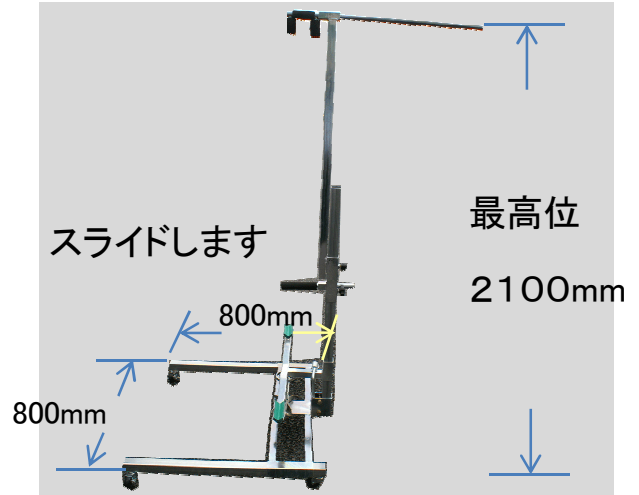
全体図
